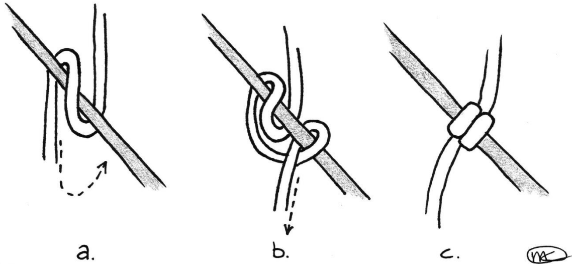
Figuur 3: De Kordonknoop (werkend naar rechts)
